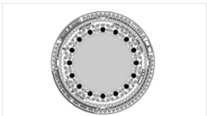
SCHACHTABDECKUNG BETON/GUSS KL.D, RUND, LW600, MIT LUFT UND EINLAGE P400011
